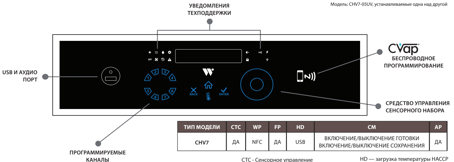
Модель: CHV7-05UV, устанавливаемые одна над другой
