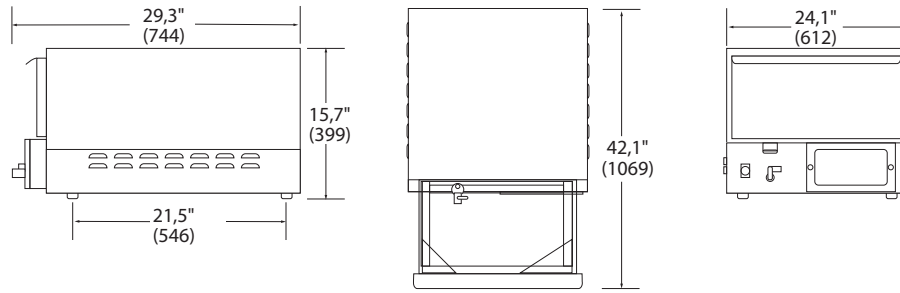
Seitenansicht
